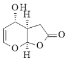
Fig. 3. Absolute configuration (4 S ,5 R ,6 R ) of oxysporone ( 1 ).
